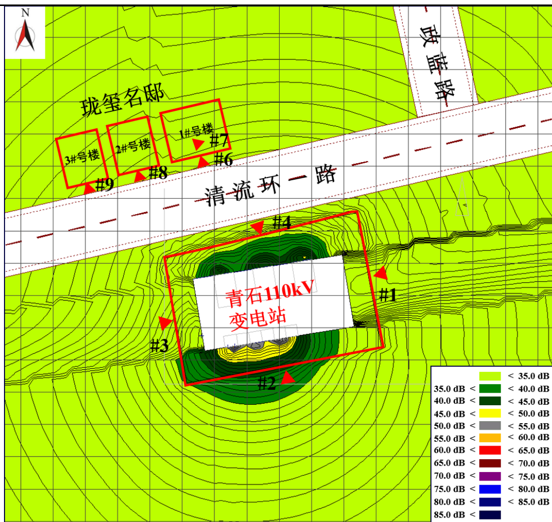
图 4.4-9 远期规模噪声影响预测结果（3m 预测高度）（图示网格线为 10m*10m） 变电站厂界噪声预测结果见表 4.4-4。
