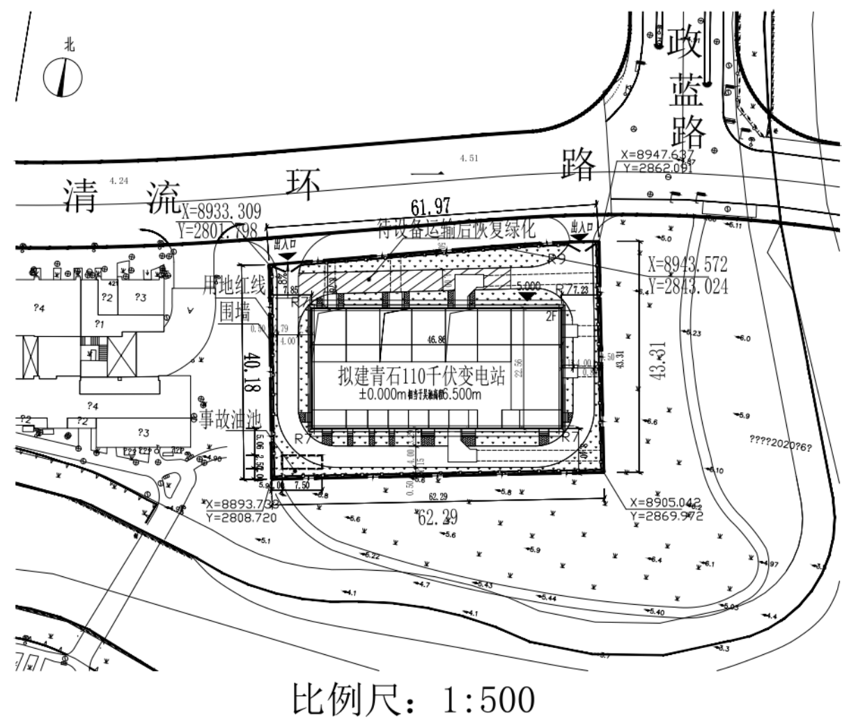
附图 4 青石 110kV 变电站总平面布置图
