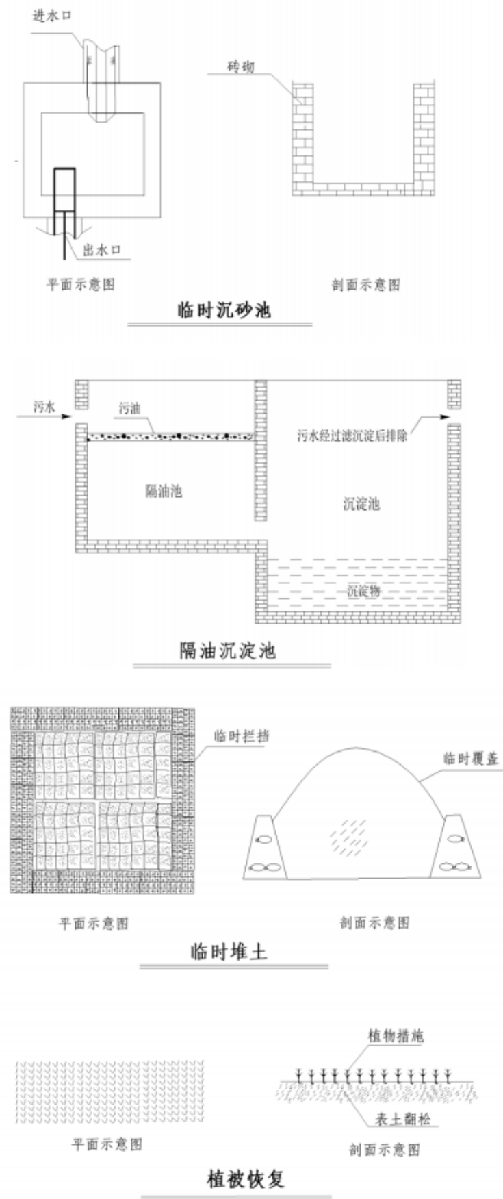
附图 14 本项目生态环境保护措施设计
