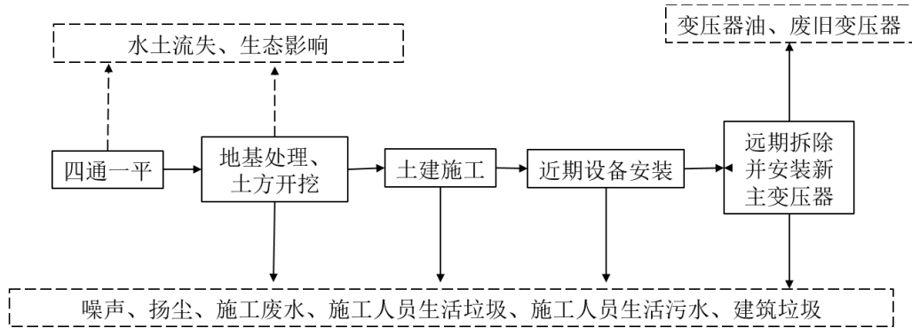
图 4.1-1 施工期工艺流程与产污环节
