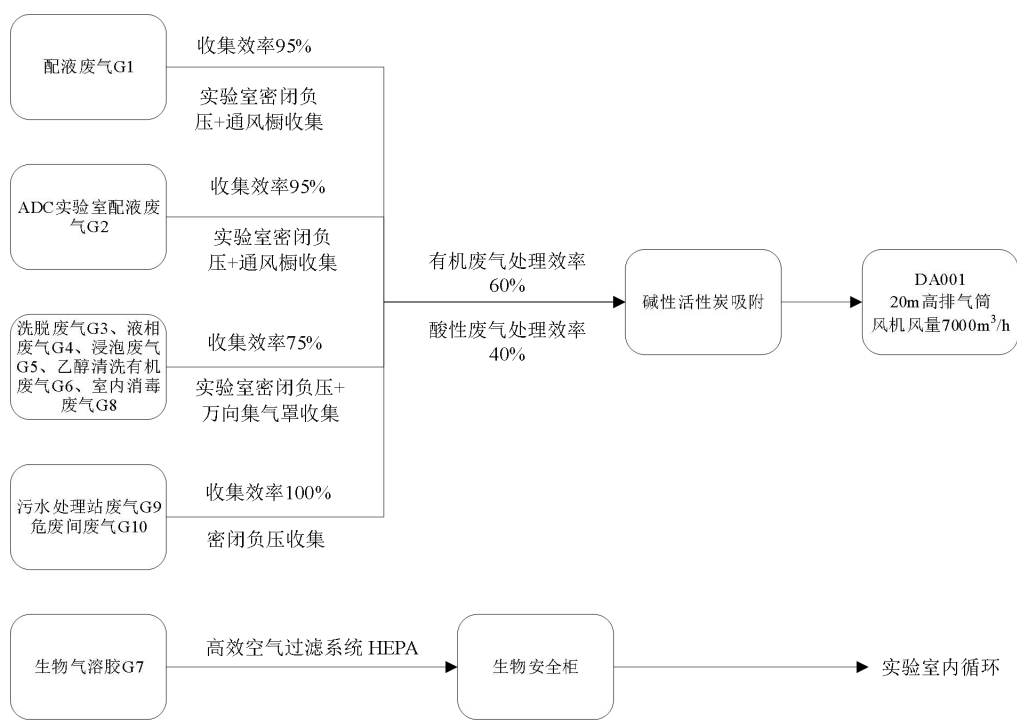
图 4-1 废气处理系统图（DA001 高度 20 米）
