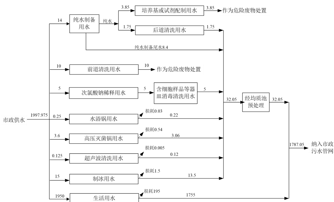
图 2-2 项目实施后全实验室水平衡图 (单位 m³/a)
