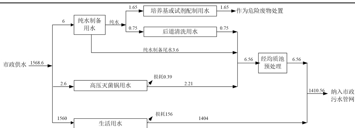
图 2-1 本项目水平衡图 (单位 m³/a)
