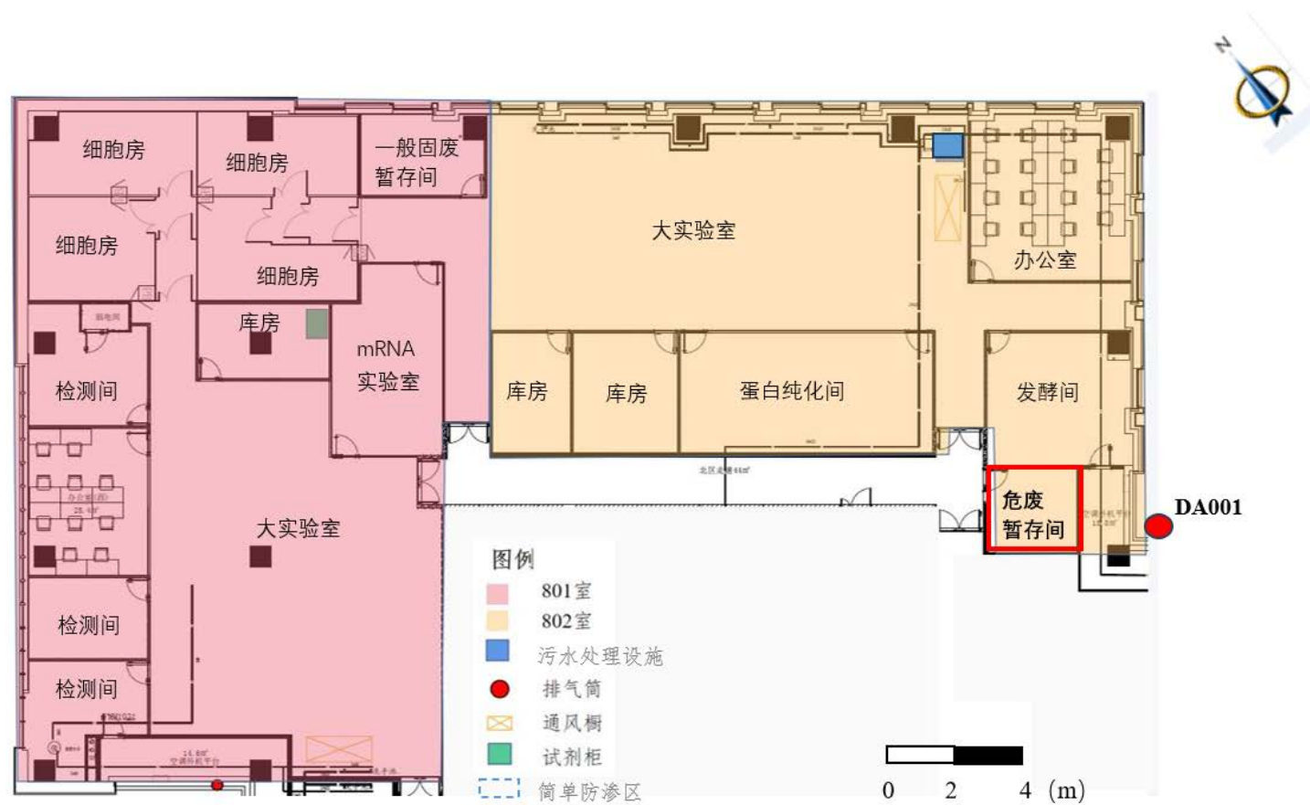
附图 4 现有项目 8 层实验室平面布置图
