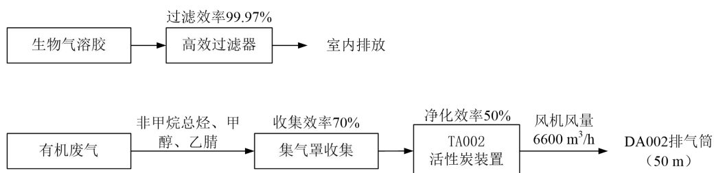
图 4-1 本项目废气收集处理措施图
