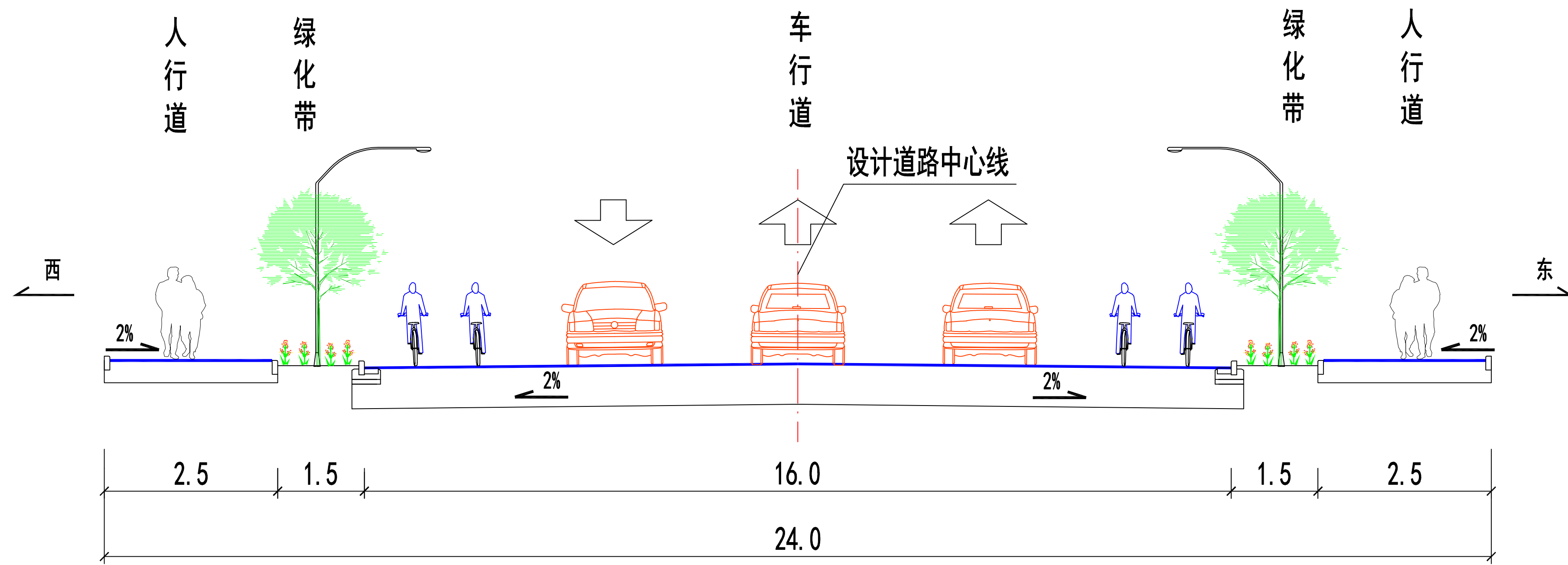
渠化段横断面设计图
