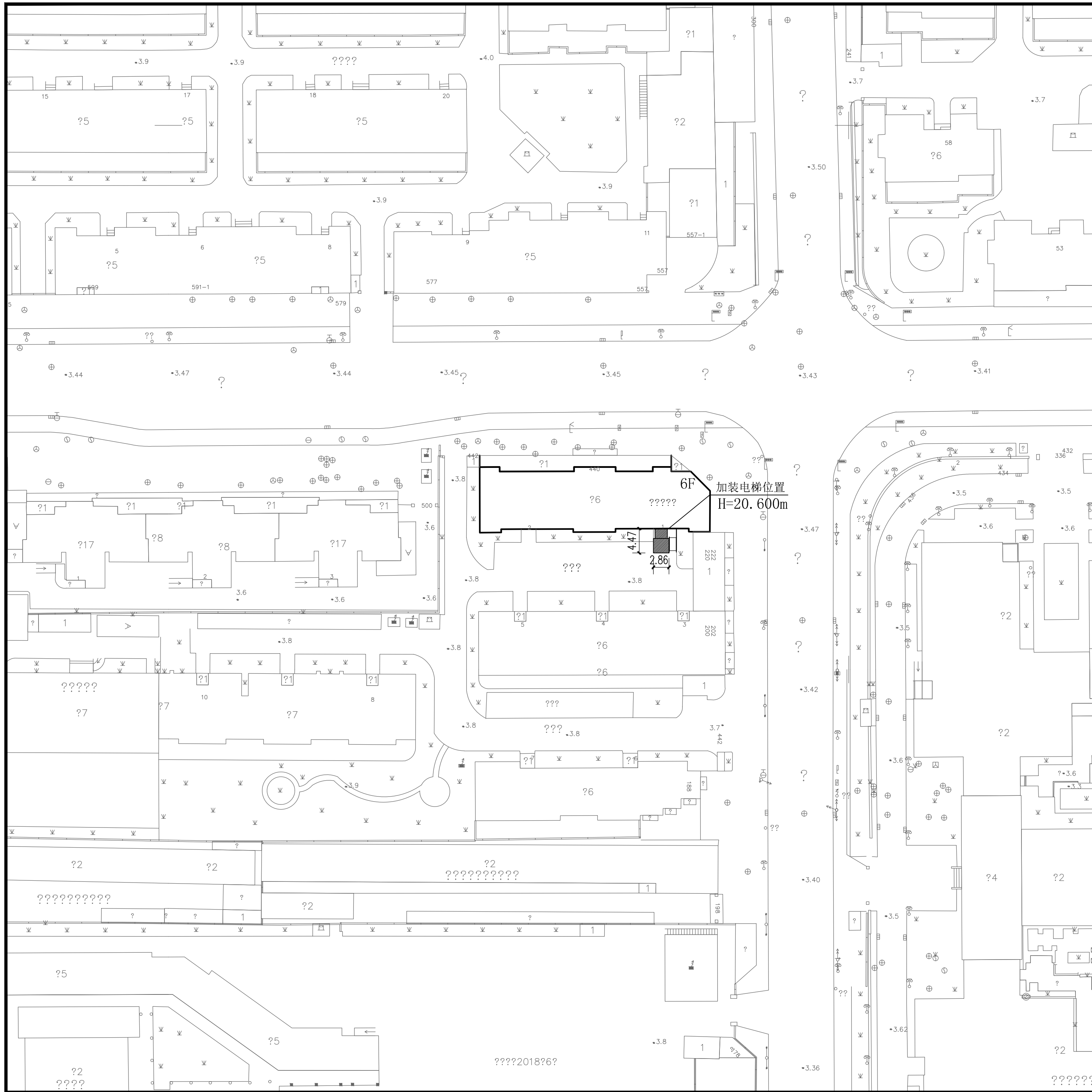
总平面图 1:500
